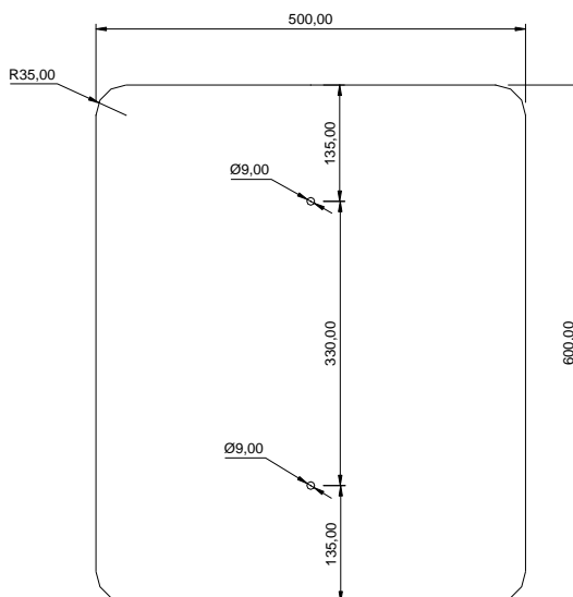
Detalhe chapa 50x60 cm – Vista frontal
