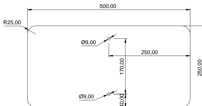
Detalhe chapa 50x25 cm – vista frontal
