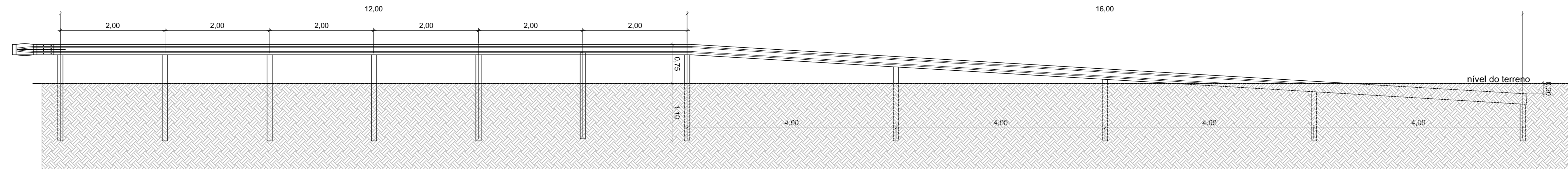
DETALHE - Guard Rail ESC. 1/50
